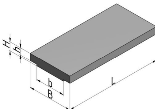
Obr. č.1 – Technický výkres zákrytové krycí destičky DK3
