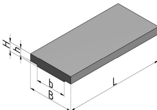
Obr. č.1 – Technický výkres zákrytové krycí destičky DK2
